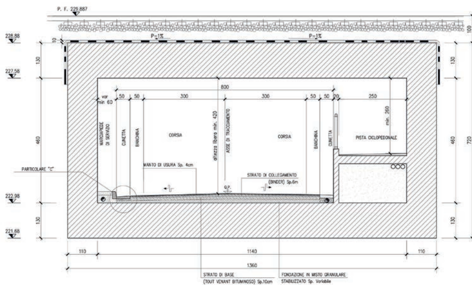
Sezione del sottopassaggio
